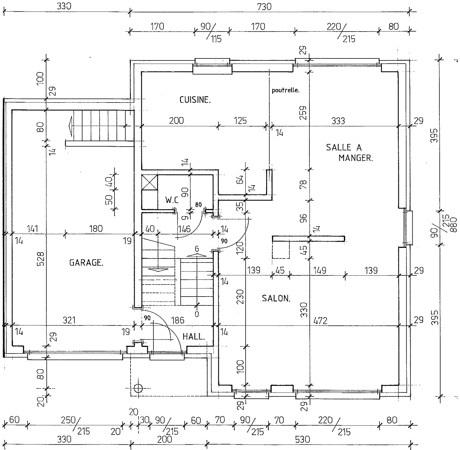
rez-de-chaussee.
